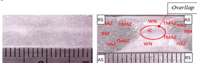
Gambar 6. a). Raw Material, b). Tanpa groove
