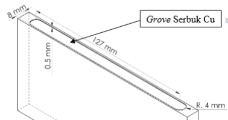
Gambar 2. Dimensi Grove Serbuk Cu
