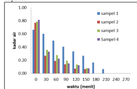
Gambar 3. Kadar air serbuk bayam yang diperoleh dari proses pengeringan dengan metode foam mat drying pada suhu 70°C dan variasi penambahan maltodekstrin 15-25%.
