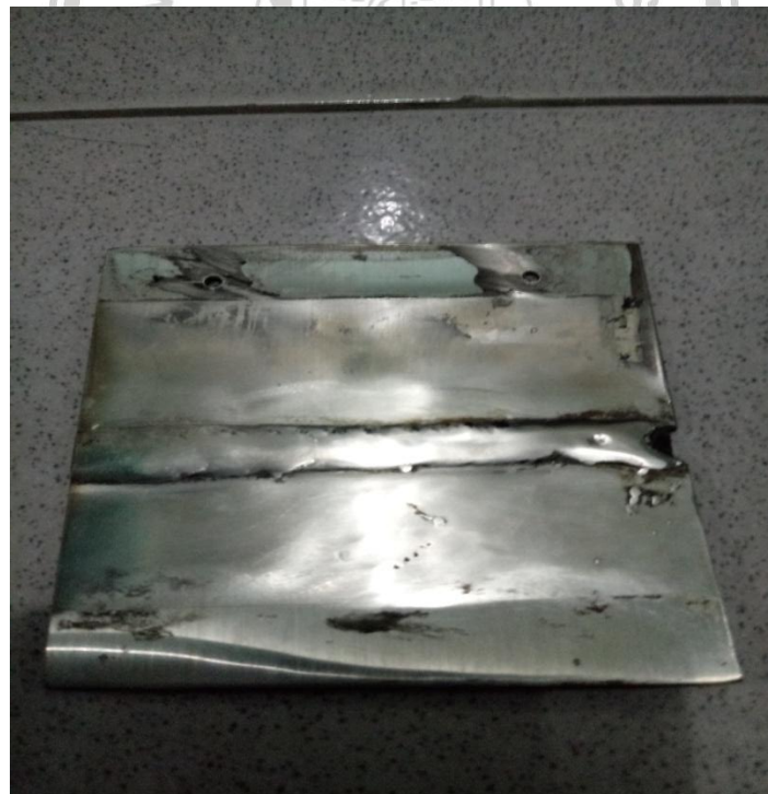
Gambar Spesimen Pengelasan SMAW Sebelum Pengujian
